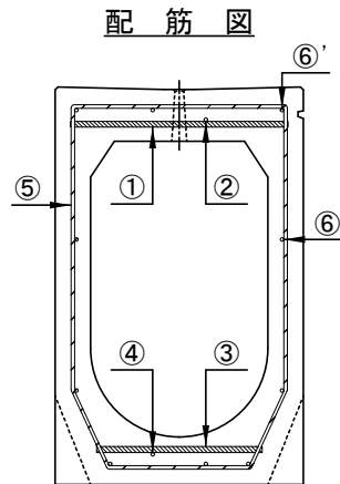
中央断面図
