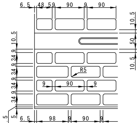
パターン詳細図
