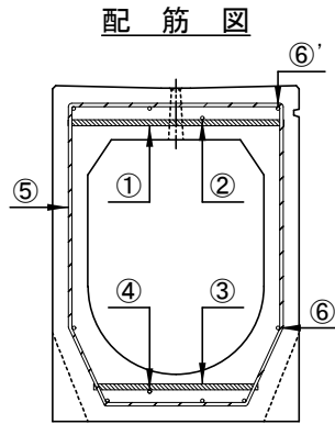
配筋図
