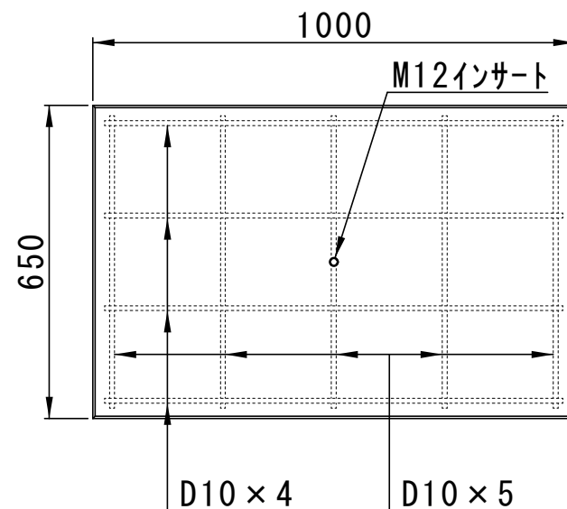
側面図
