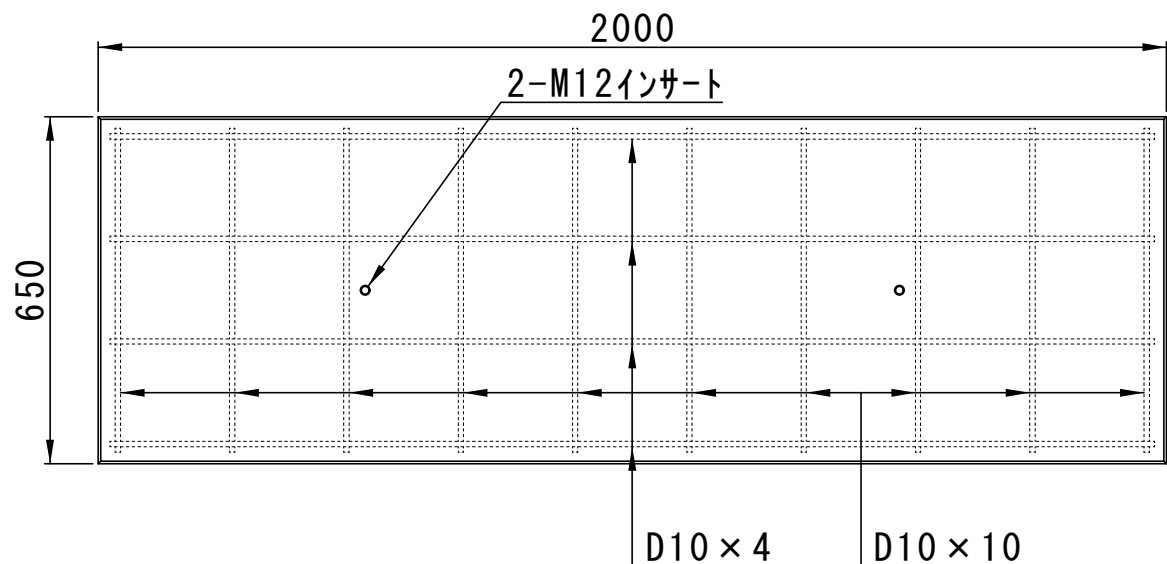
平面図
