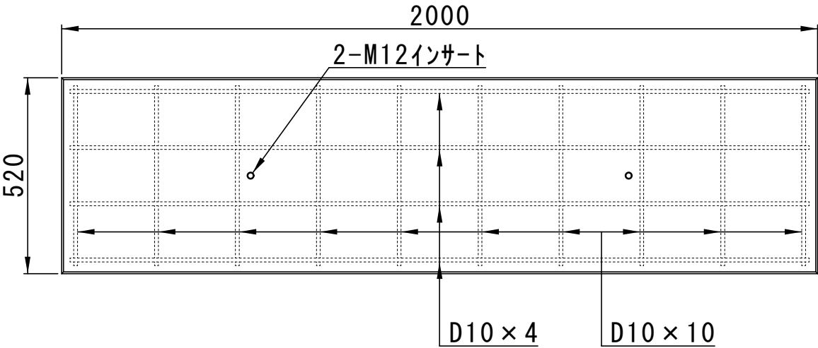
平面図
