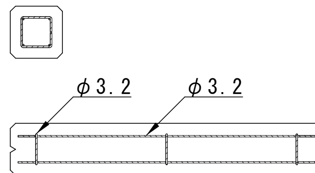
配筋図
