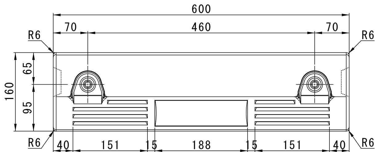
平面図
