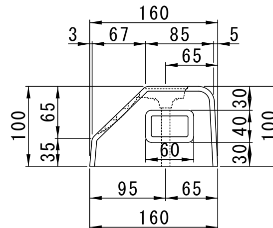
側面図
