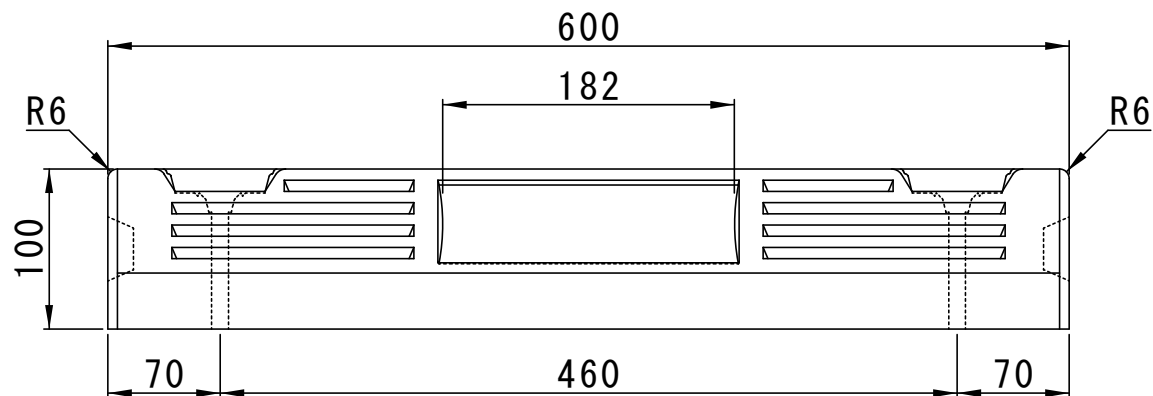
正面図
