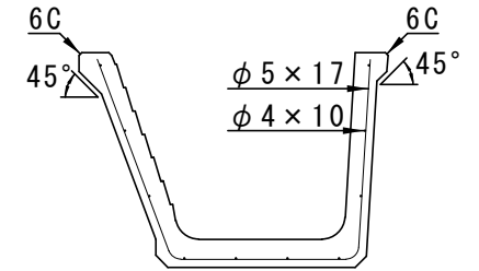
配筋図
