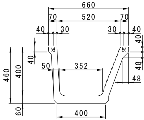
中央断面図
