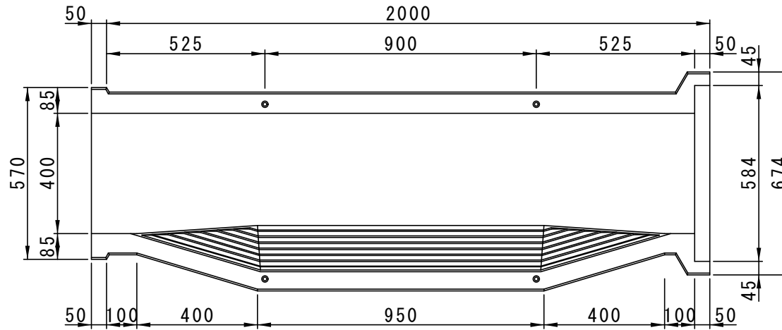
平面図
