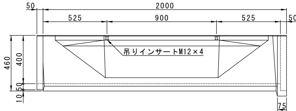
側面図
