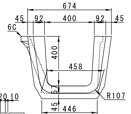
背面図
