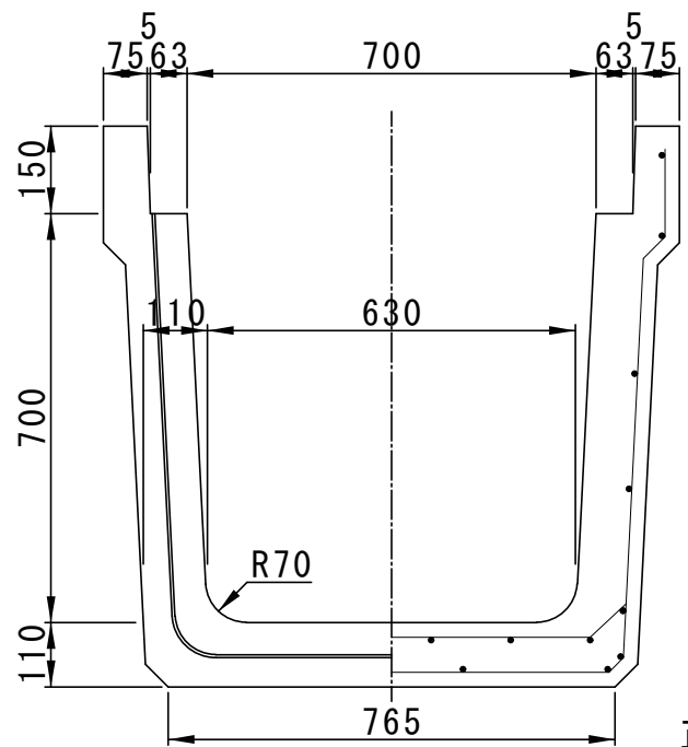
正面図
