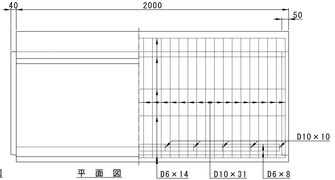
側面図 本体参考重量 1,300kg
