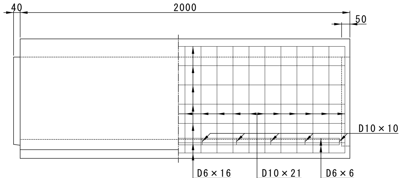
側面図
