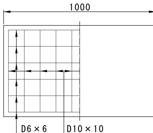
平面図
