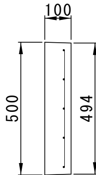
正面図
