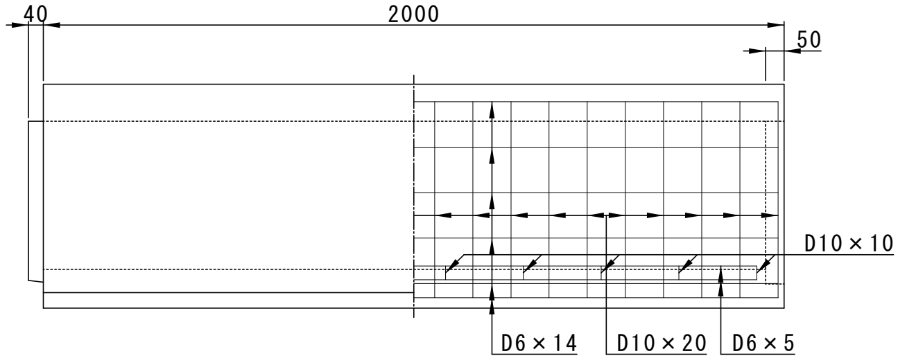
側面図
