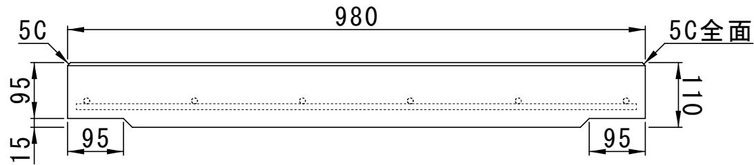
平面図
