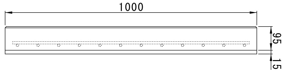
側面図
