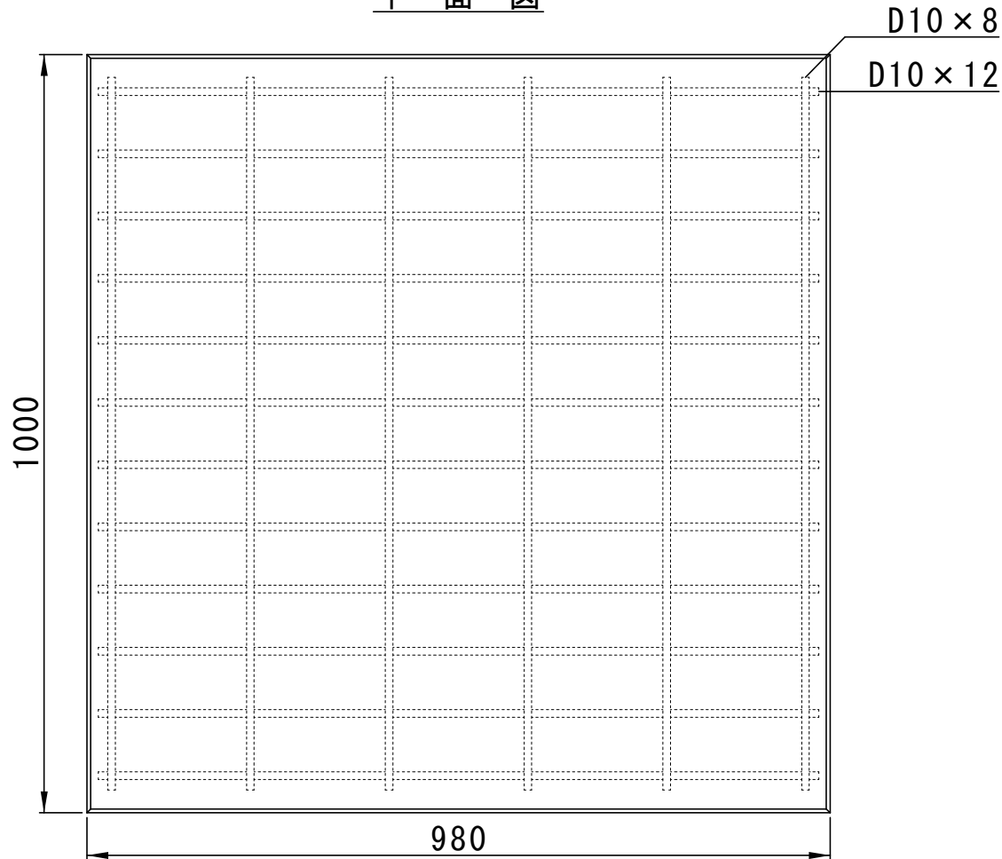
平面図
