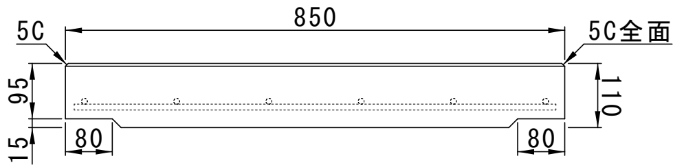
平面図
