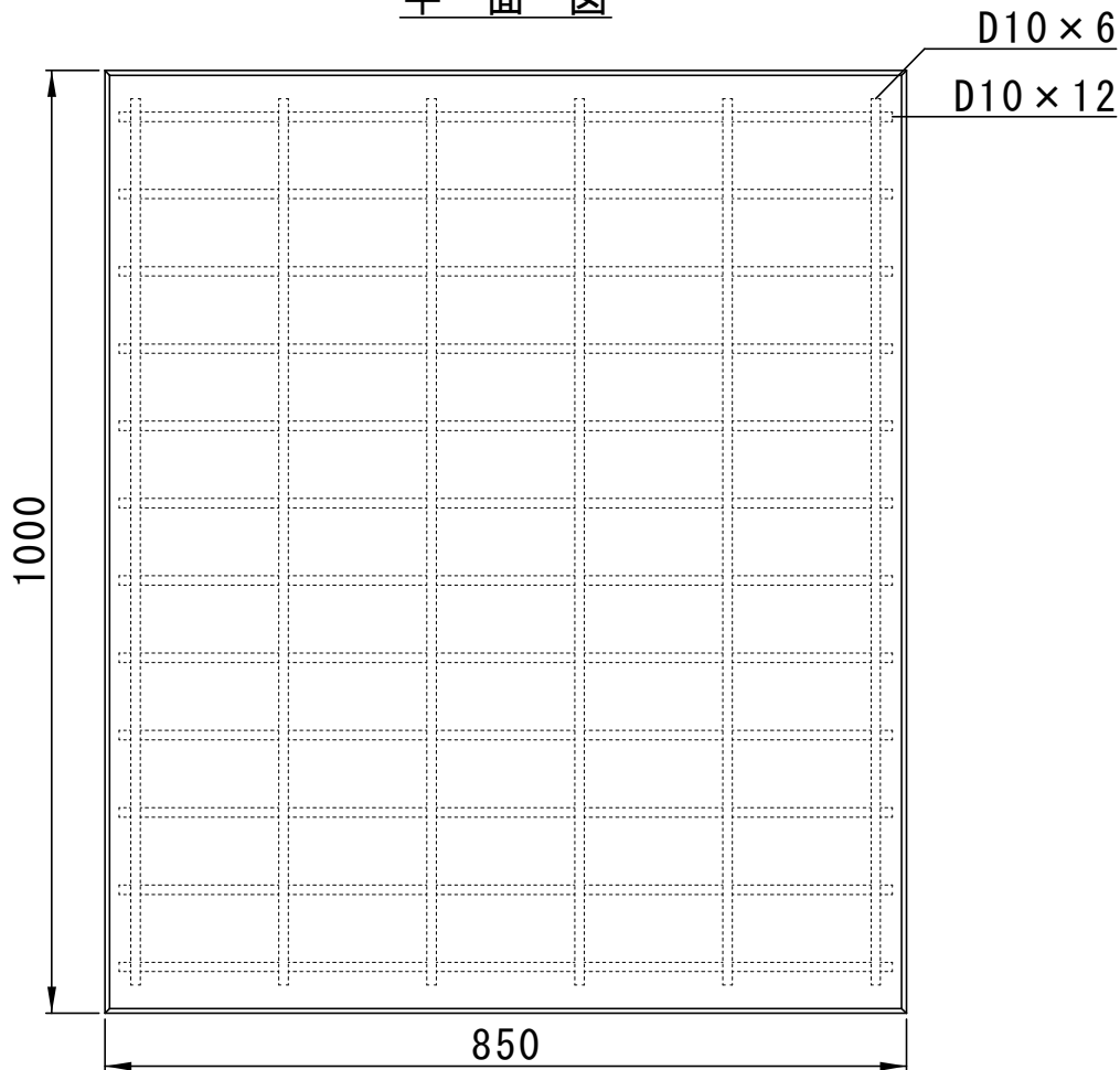
平面図
