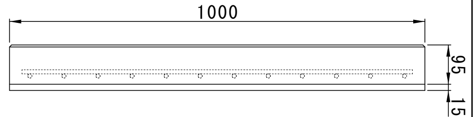
側面図
