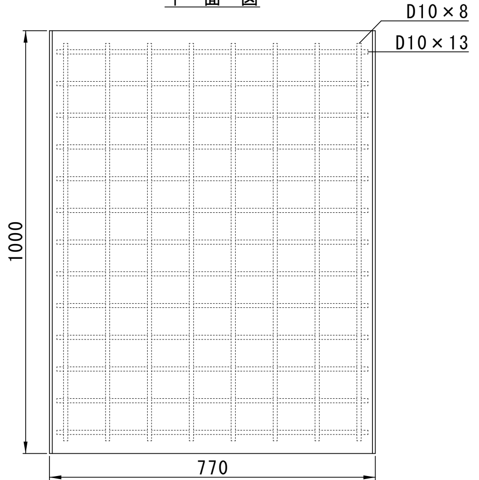
平面図
