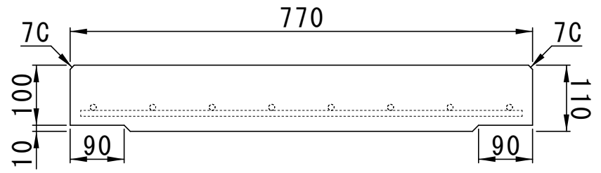
平面図
