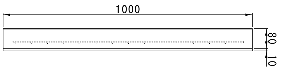
側面図
