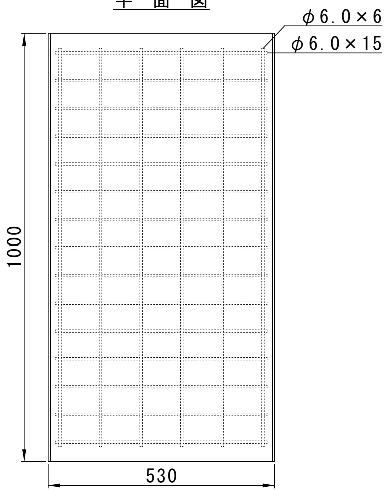
平面図
