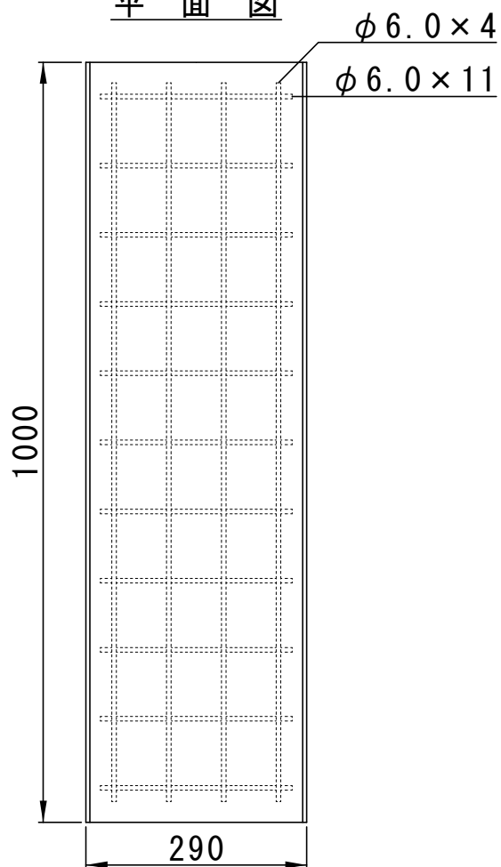
平面図
