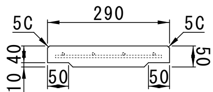
正面図
