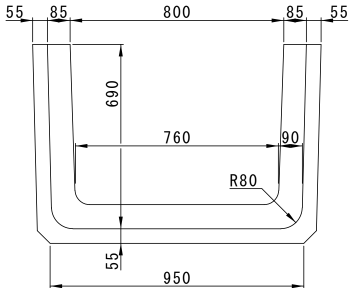
A-A' 断面
