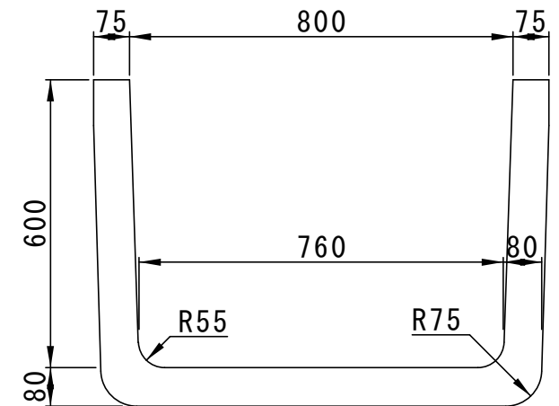
C-C' 断面
