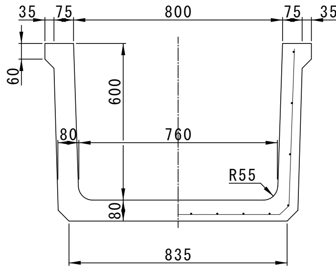
B-B' 断面
