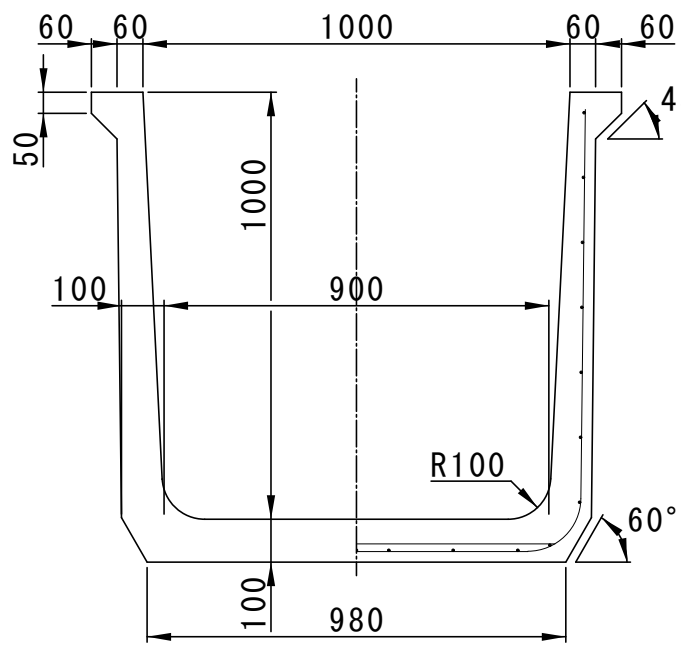
B-B' 断面
