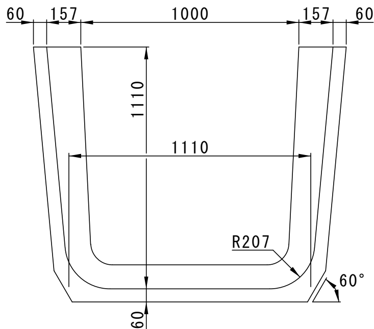
A-A' 断面
