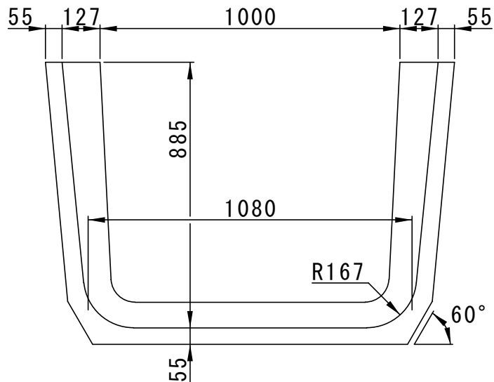
A-A' 断面
