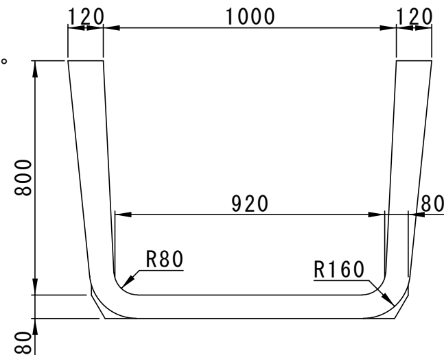
C-C' 断面
