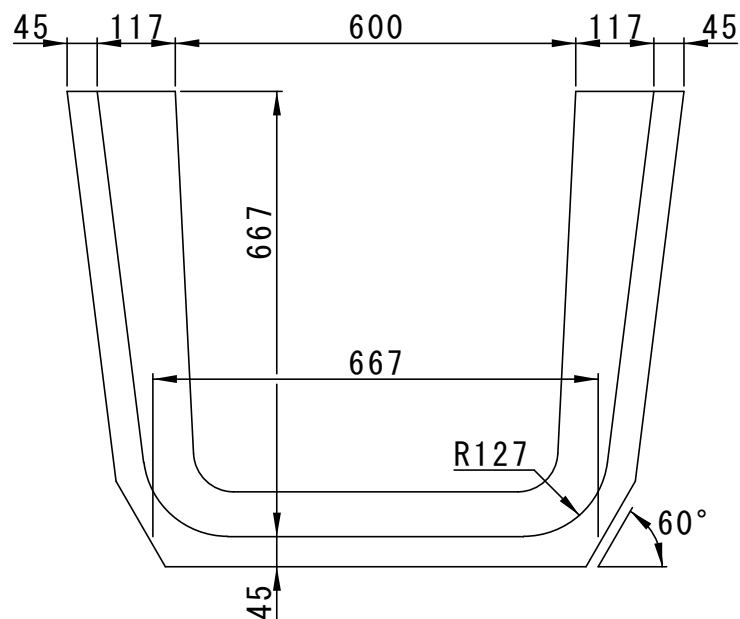
A-A' 断面
