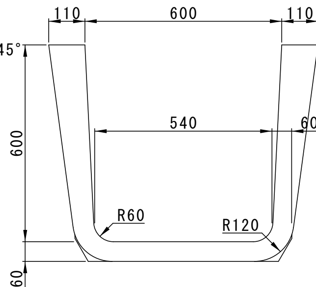
C-C' 断面
