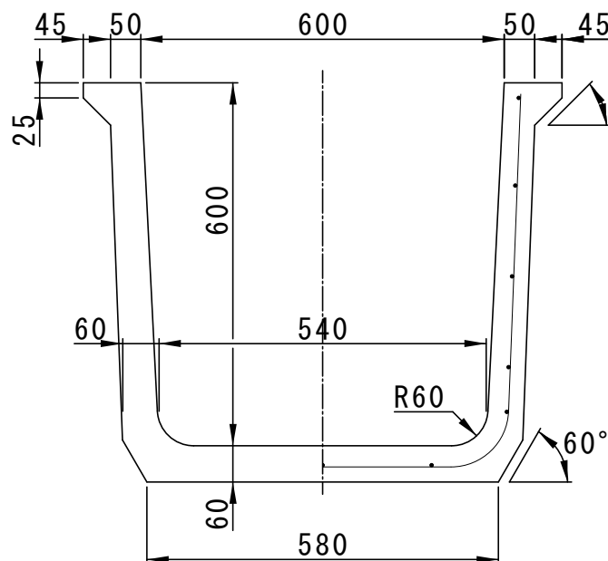
B-B' 断面
