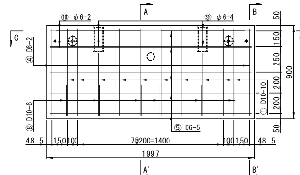
配筋図(縦壁)
