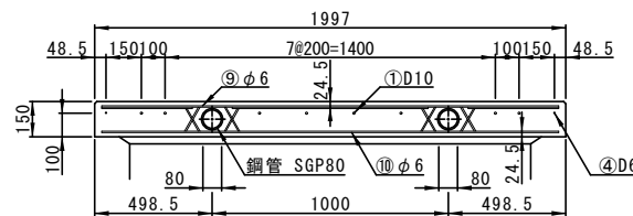
縦壁断面図詳細(C-C')
