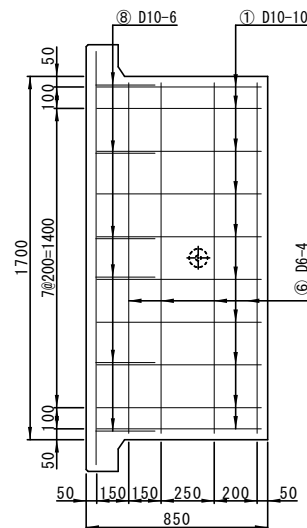
配筋図(底板)
