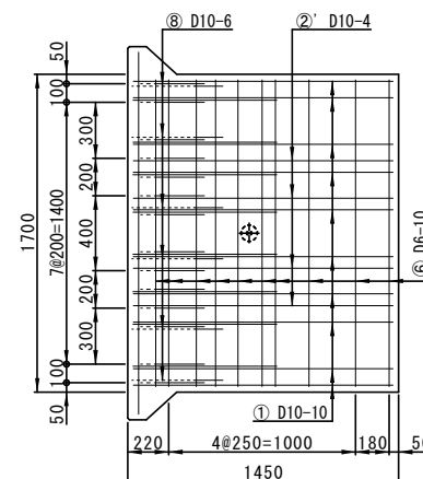
配筋図(底板)
