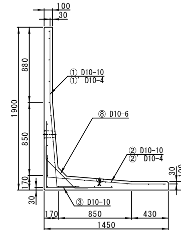
配筋図(側面A-A')
