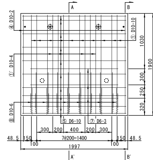
配筋図(縦壁)
