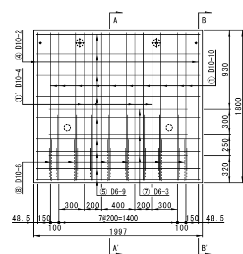
配筋図(豎壁)
