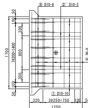
配筋図(底版)
