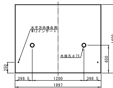
正面図
