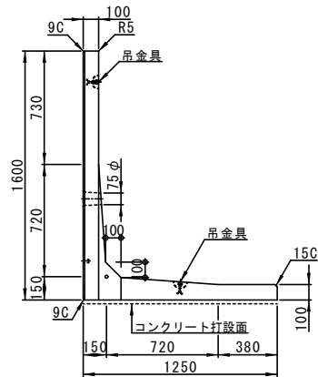
側面図
