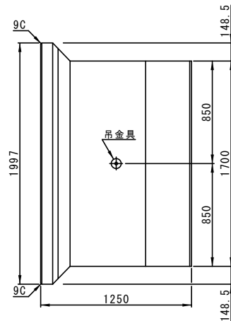
平面図
