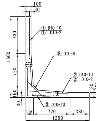
配筋図(側面A-A')
