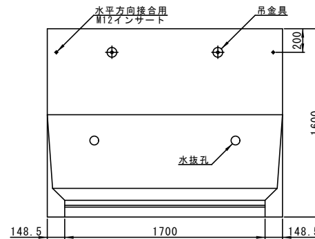
背面図
