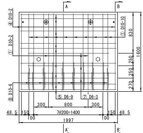
配筋図(縦壁)
