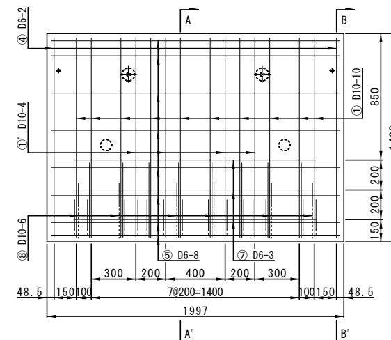
配筋図(豎壁)
