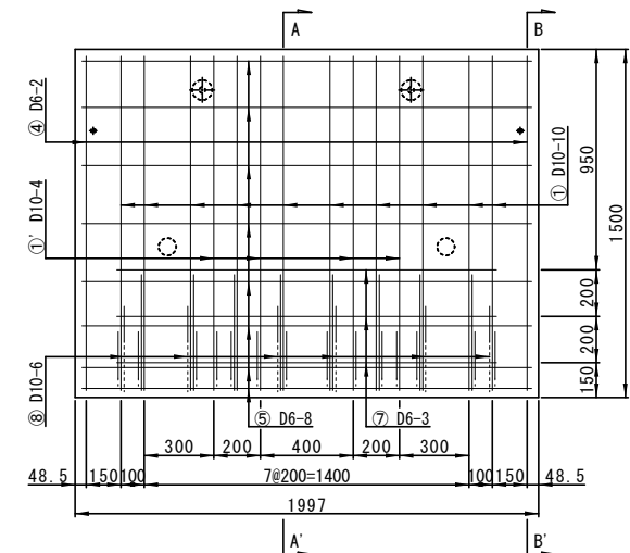
配筋図(縦壁)
