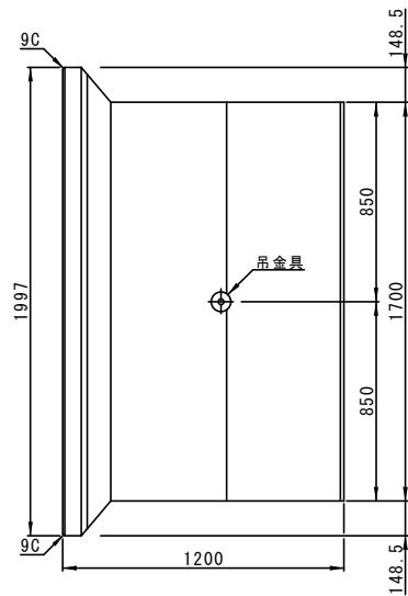
平面図
