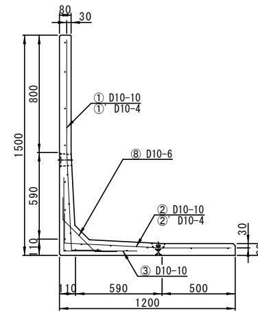
配筋図(側面A-A')
