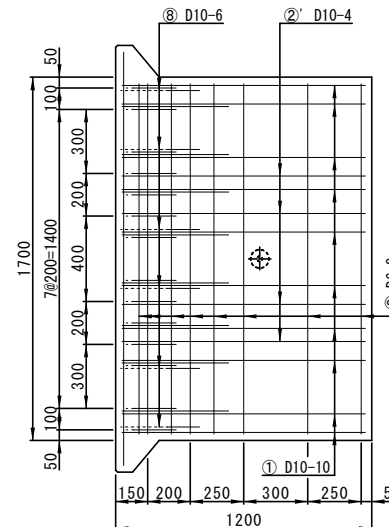
配筋図(底版)
