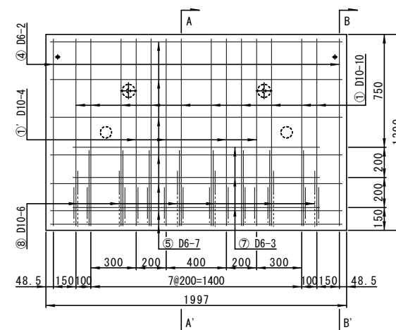
配筋図(縦壁)
