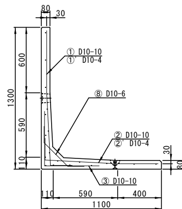
配筋図(側面A-A')
