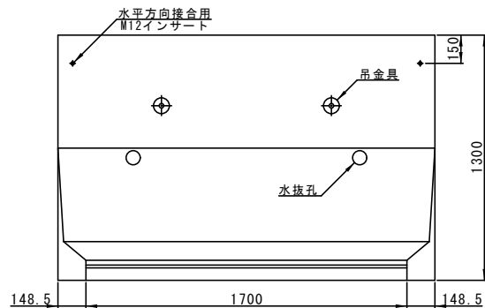
背面図
