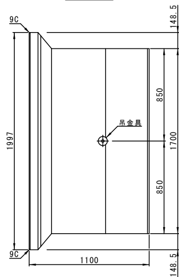
平面図
