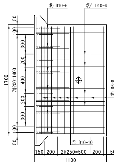
配筋図(底板)
