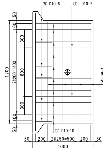
配筋図(底版)
