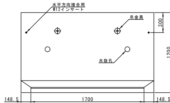
背面図
