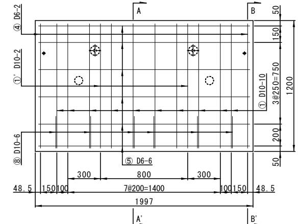
配筋図(縦壁)
