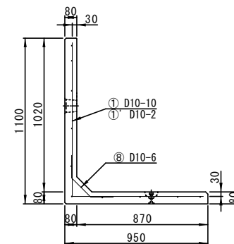
配筋図(側面A-A')
