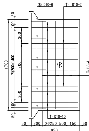
配筋図(底板)
