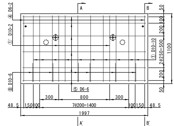
配筋図(縦壁)
