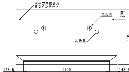
背面図
