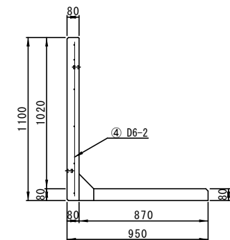
配筋図(側面B-B')
