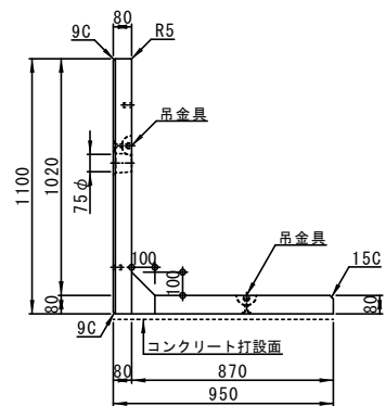
側面図
