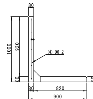
配筋図(側面B-B')
