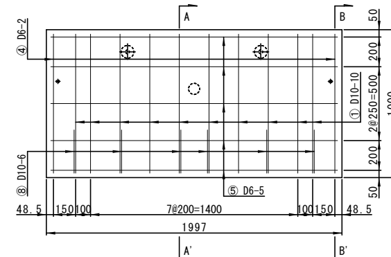
配筋図(壁壁)
