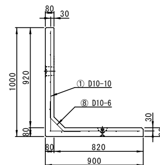
配筋図(側面A-A')
