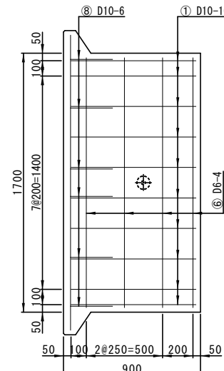
配筋図(底版)
