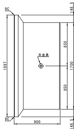
平面図
