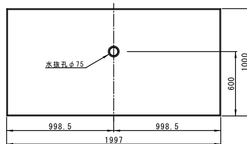
正面図
