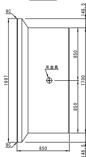
平面図
