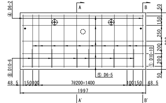
配筋図(縦壁)
