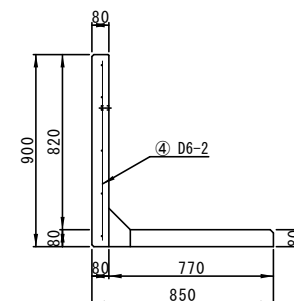
配筋図(側面B-B')
