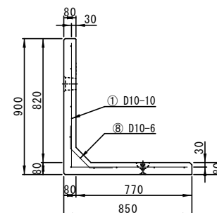
配筋図(側面A-A')
