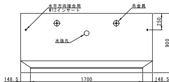
背面図
