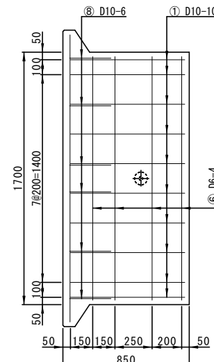
配筋図(底板)
