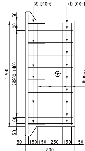
配筋図(底版)
