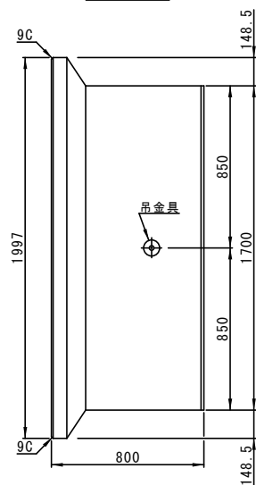
平面図
