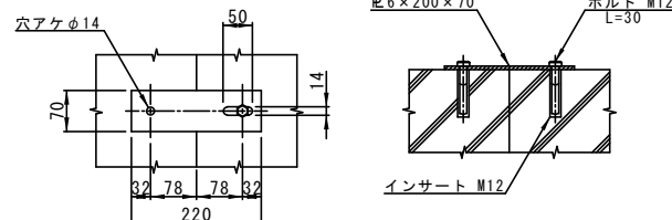
継手金具詳細図 S=1/11
