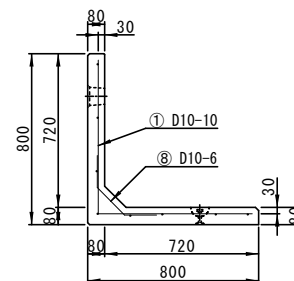
配筋図(側面A-A')
