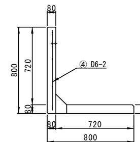
配筋図(側面B-B')
