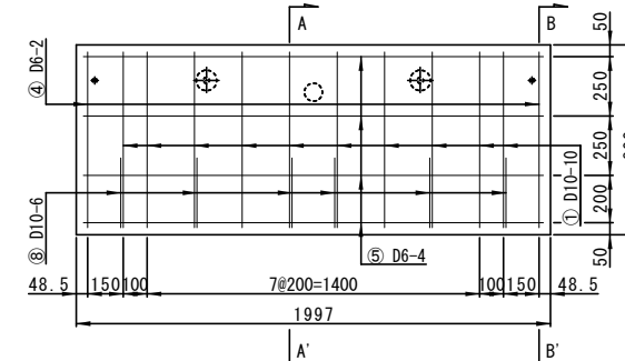
配筋図(縦壁)
