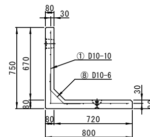
配筋図(側面A-A')
