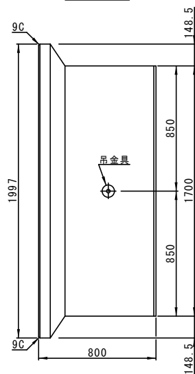
平面図
