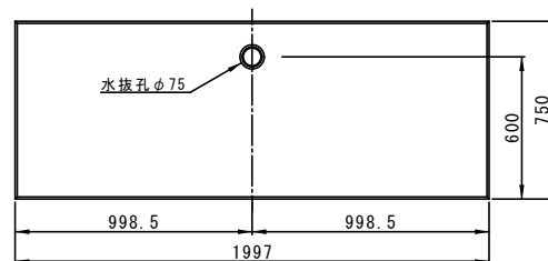
正面図
