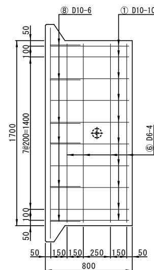
配筋図(底版)
