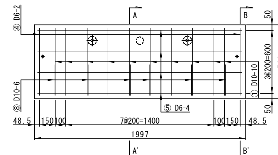
配筋図(縦壁)
