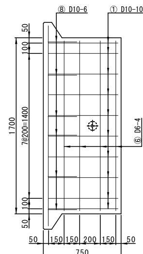
配筋図(底版)
