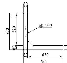
配筋図(側面B-B')
