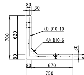
配筋図(側面A-A')
