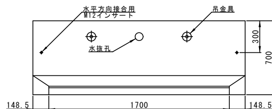
背面図
