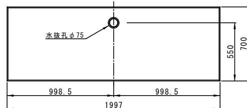
正面図
