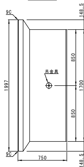
平面図
