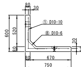
配筋図(側面A-A')
