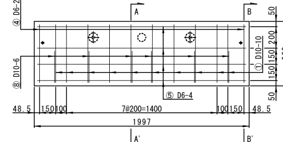
配筋図(縦壁)
