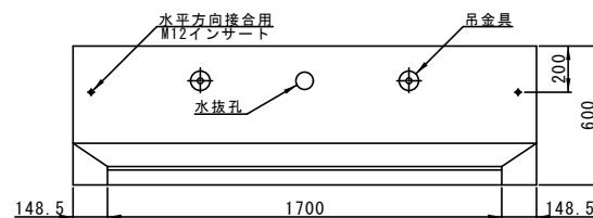
背面図
