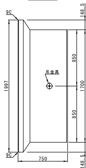
平面図
