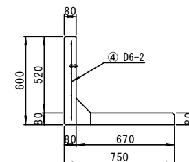
配筋図(側面B-B')
