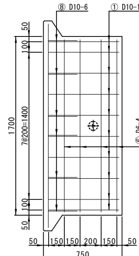
配筋図(底板)
