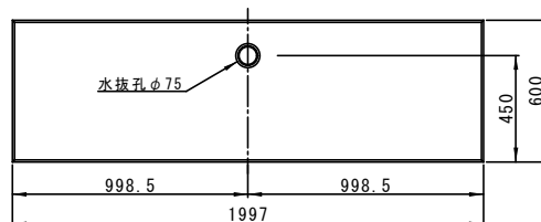
正面図
