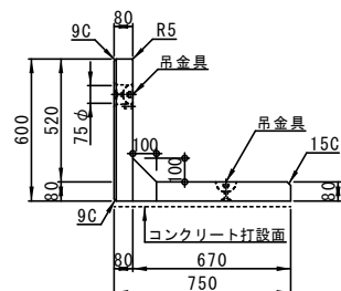
側面図
