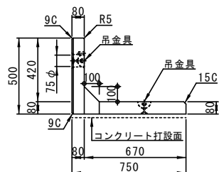
側面図
