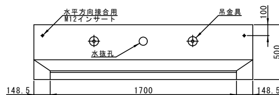
背面図
