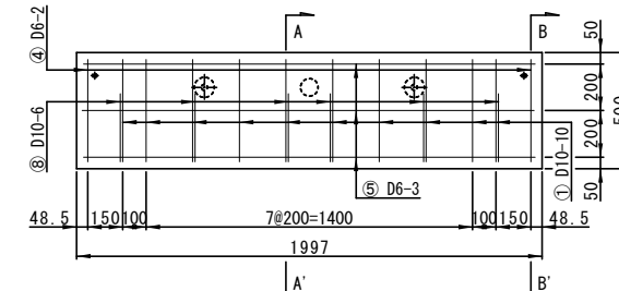
配筋図(縦壁)
