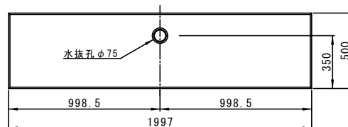
正面図
