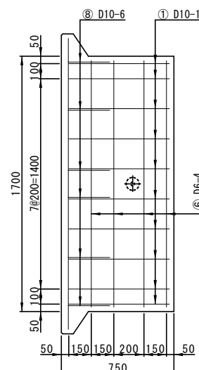
配筋図(底版)
