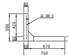
配筋図(側面B-B')
