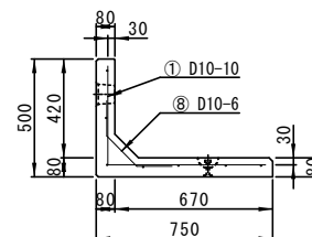
配筋図(側面A-A')
