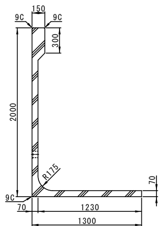
断面 A-A'
