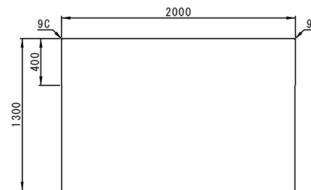
底板 (下面)
