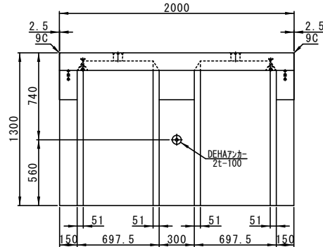
底板 (上面)
