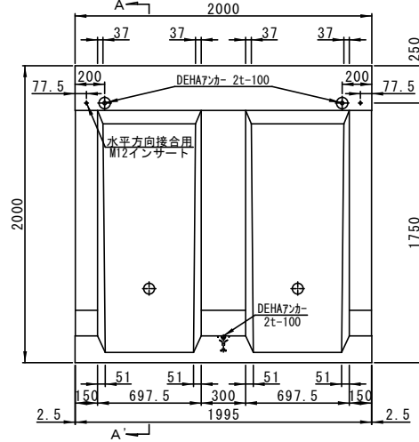
縦壁 (背面)
