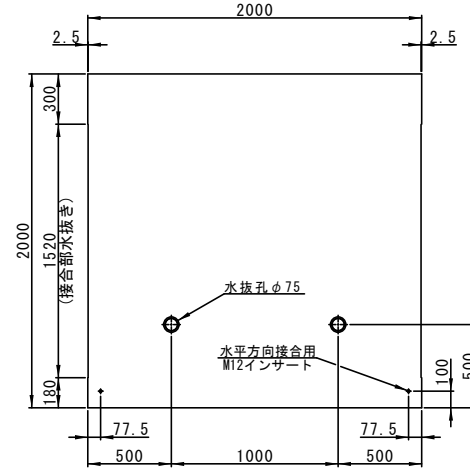
縦壁 (前面)
