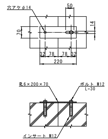
継手金具詳細図 S=1/11
