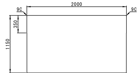
底板(下面)
