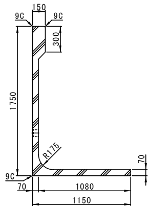
断面A-A'
