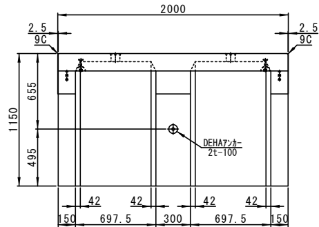
底板(上面)
