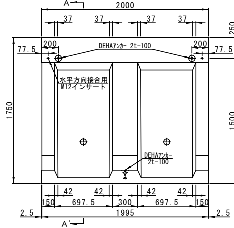
縦壁(背面)
