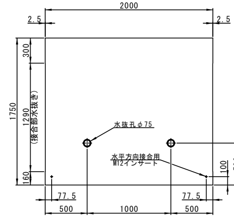
縦壁(前面)
