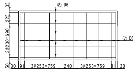
底板(下面)
