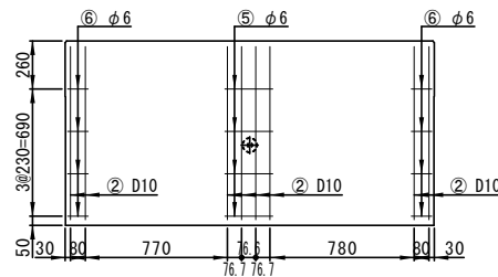
底板(上面)
