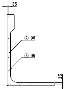
断面B-B'
