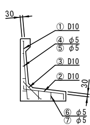
断面A-A'
