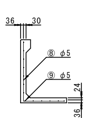
断面B-B'
