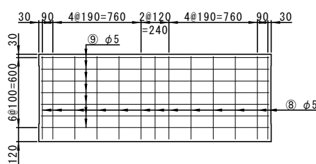
堅壁(前面)
