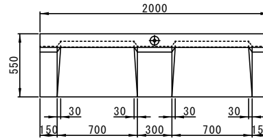
底版(上面)
