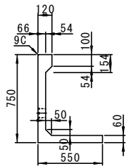
断面B-B'
