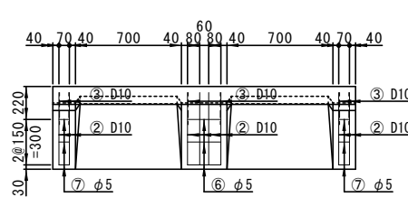
底版(上面)
