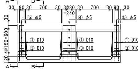
堅壁(背面)
