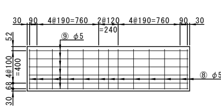
底版(下面)
