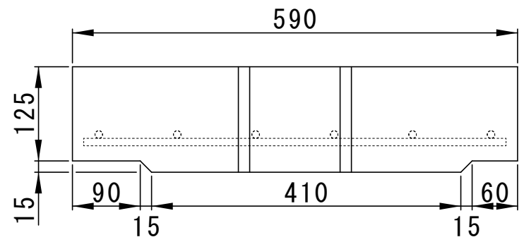
正面図
