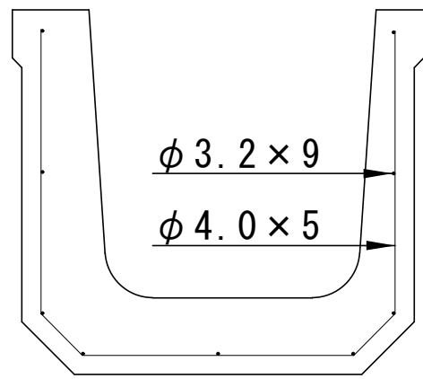
配筋図
