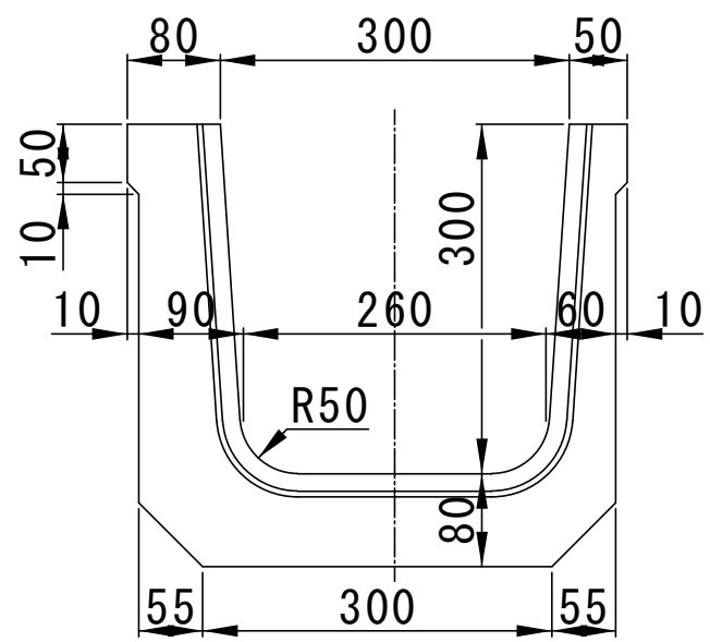
正面図
