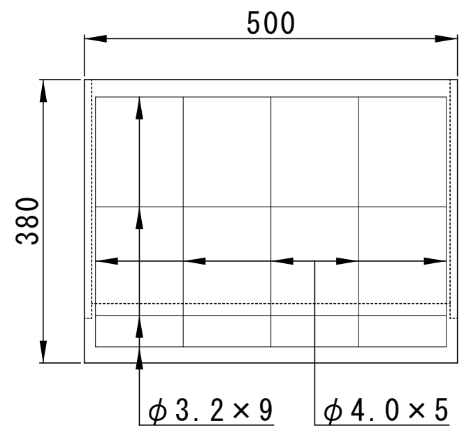
側面図
