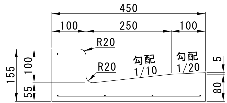
正面図
