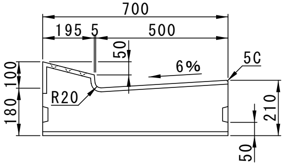
正面図
