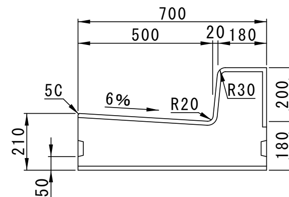
背面図
