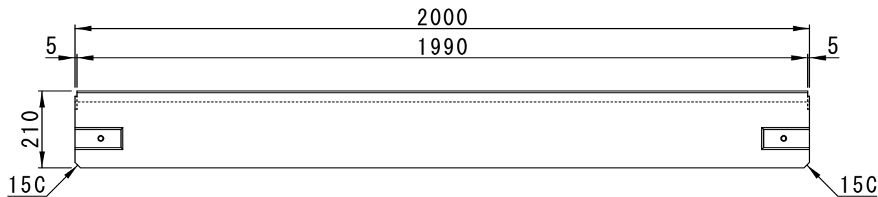
側面図
