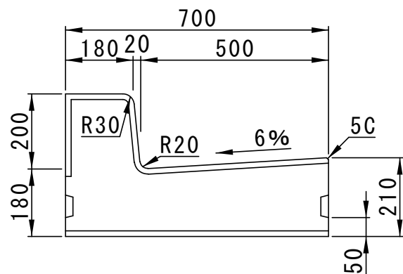
正面図
