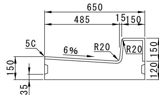
背面図
