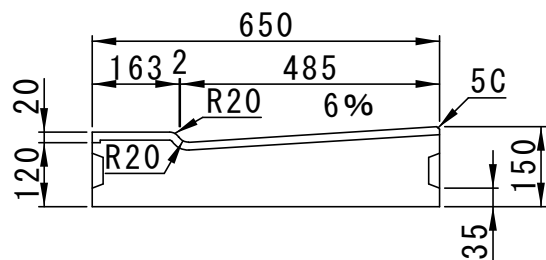
正面図
