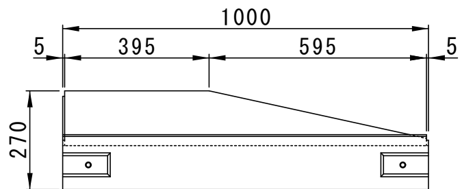
側面図
