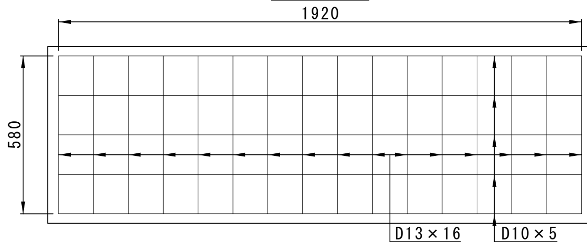
側面図
