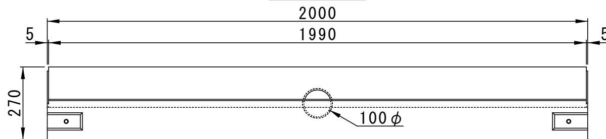
側面図
