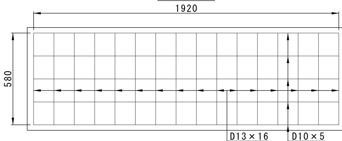
配筋図
