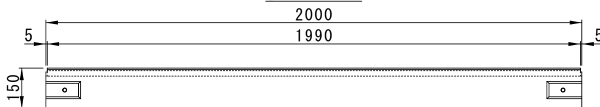
側面図
